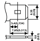
F2 (Faston Tab 250)
